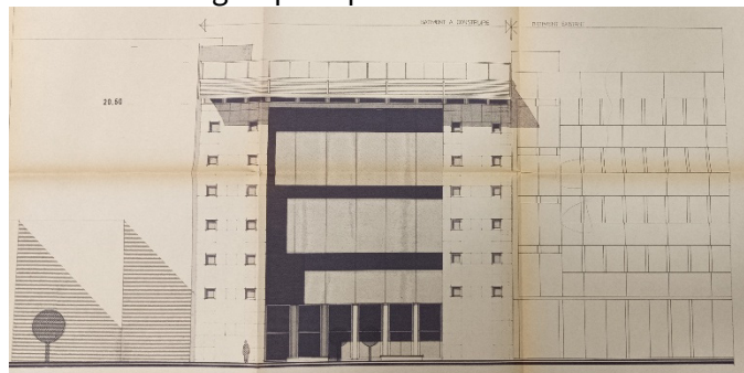
Plan d'Avant-Projet Sommaire du CRDA – façade ouest – 25/03/1991 © Service Archives MOM
